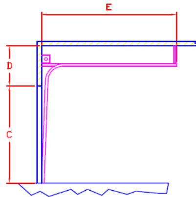
PUERTA MANUAL
